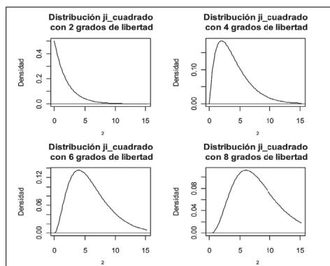
Figura 4. Distribuciones ji-cuadrado para distintos grados de libertad. Hechas en R 22
