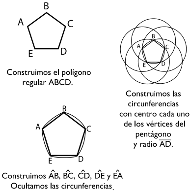
Figura 5. Pentágono de ancho constante
