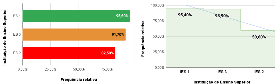
Figura 1. Desempenho no teste de Biomoléculas Fósseis por IES: (A) Média geral da taxa de acertos; (B) Análise conjunta das categorias de notas altas e médias (n=72).
