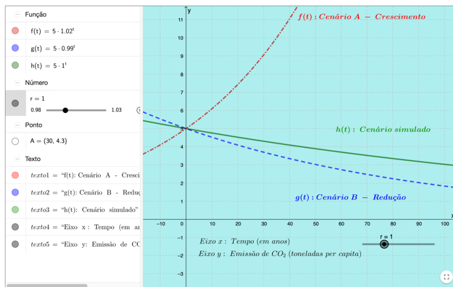
Figura 1. Modelagem matemática dos possíveis cenários da emissão de CO 2 per capita.
