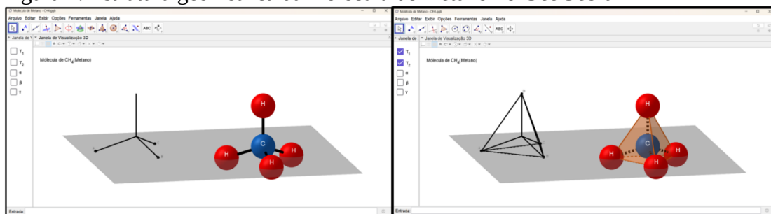
Figura 1. Estrutura geométrica da molécula de metano no GeoGebra
