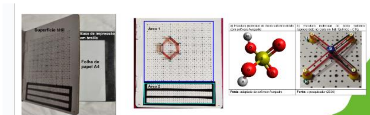
Figura 1. Caderno Tátil Químico utilizado para a representação do benzeno
