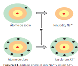
Figura 61. Enlace entre el i n \text{Na}^+ y el i n \text{Cl}^- .
